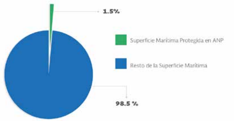
Gráfico 2. Superficie protegida respecto a territorio Marítimo Nacional.
