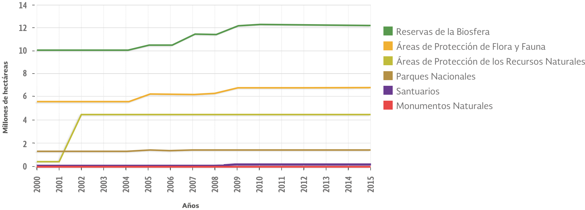
Gráfico 6. Superficie protegida acumulada a lo largo del tiempo según categoría de manejo.
