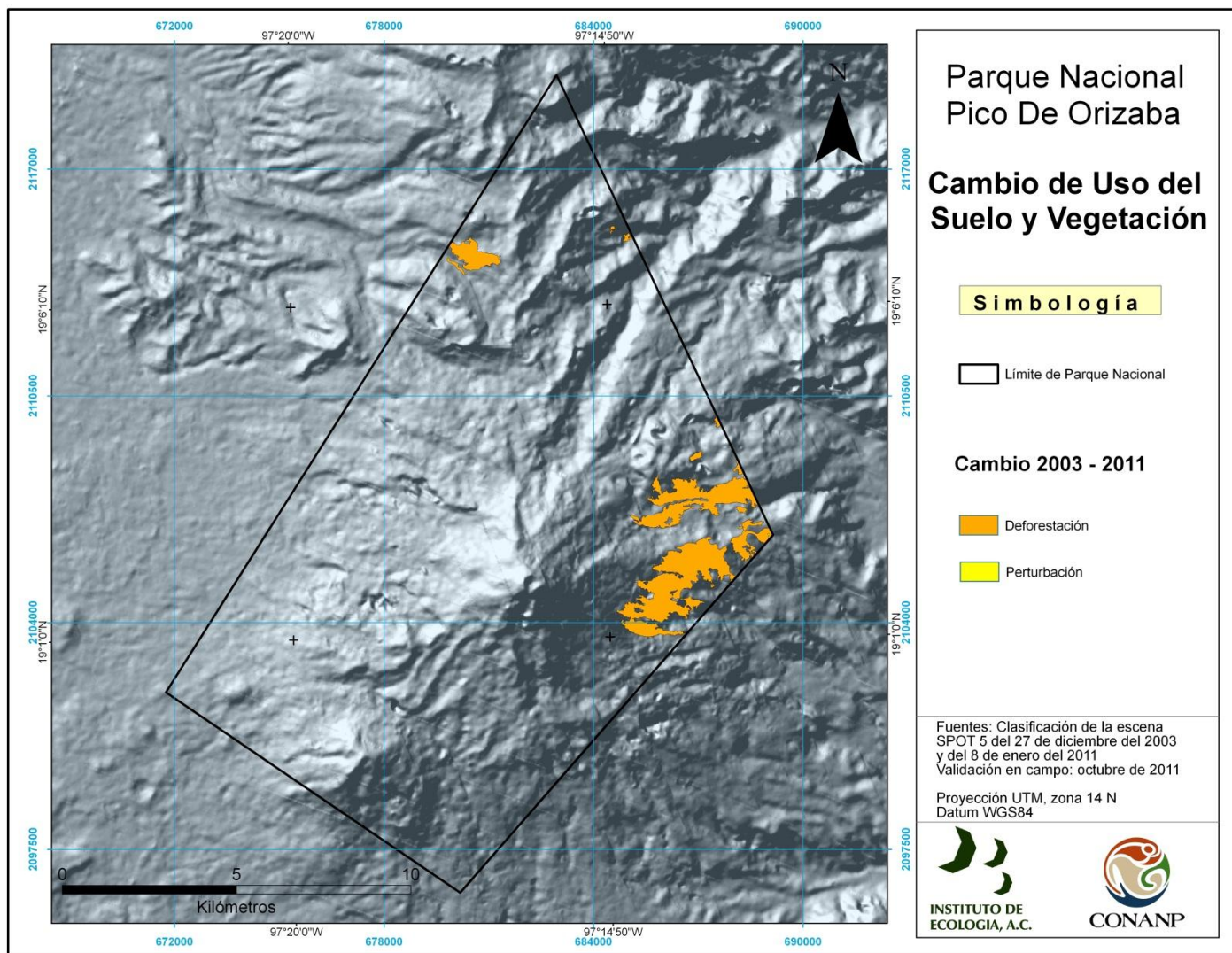
Figura 10. Cambios en el periodo 2003–2011 en el PNPO.
