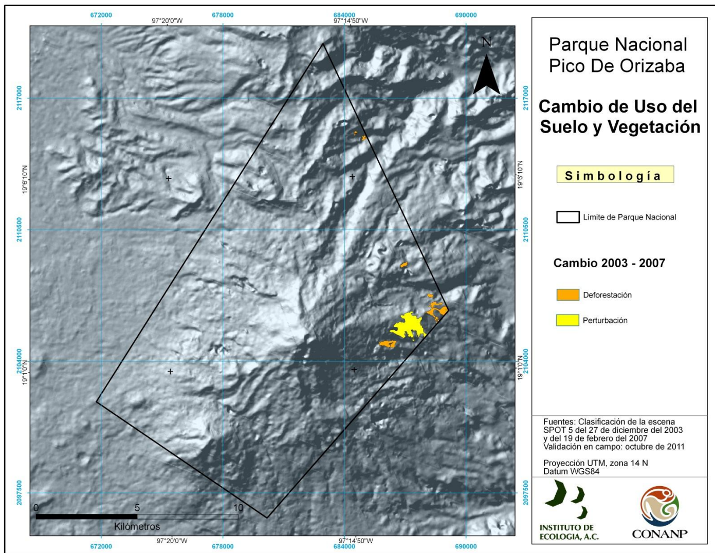
Figura 8. Cambios en el periodo 2003–2007 en el PNPO.
