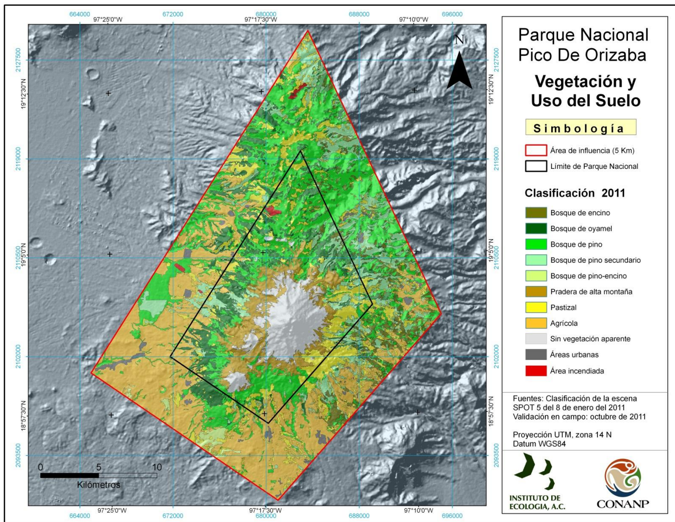
Figura 6. Imagen clasificada del año 2011.
