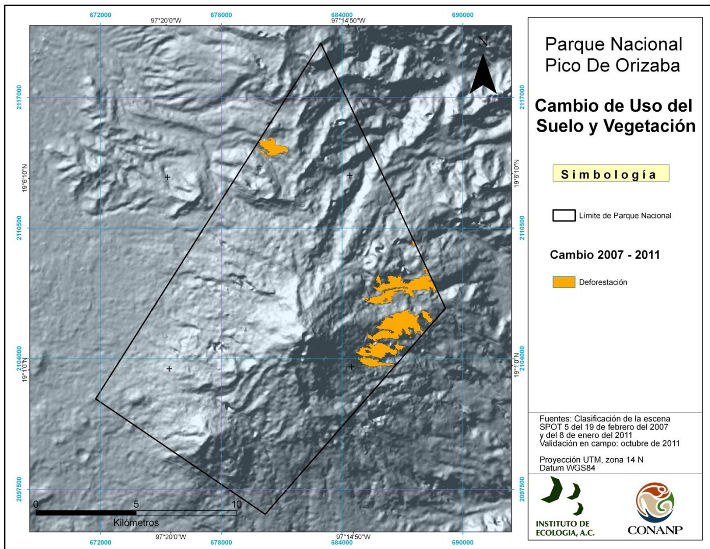
Figura 9. Cambios en el periodo 2007–2011 en el PNPO
