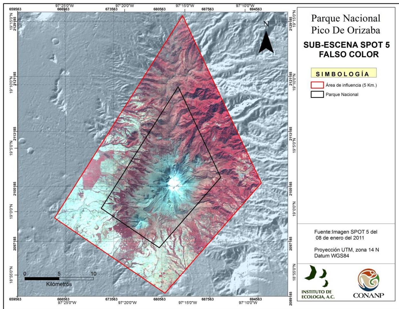
Figura 3. Sub-escena SPOT 5 del año 2011 en falso color (3, 2, 1).
