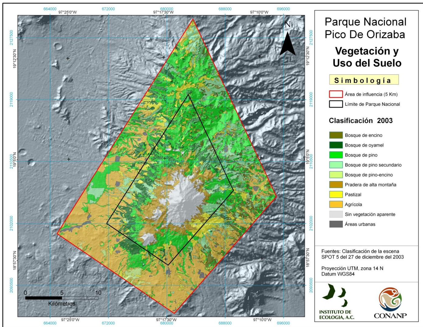
Figura 4. Imagen clasificada del año 2003
