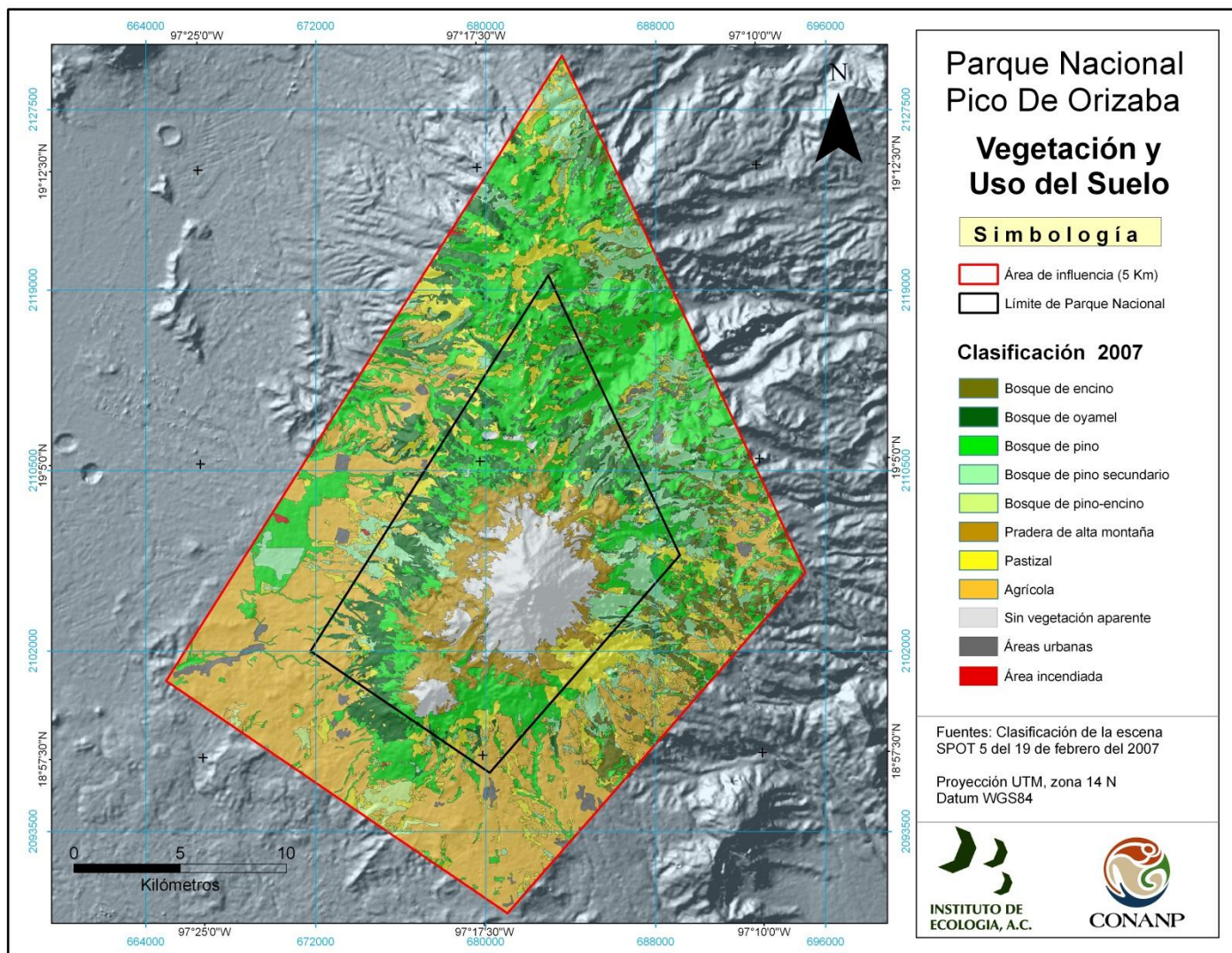
Figura 5. Imagen clasificada del año 2007.
