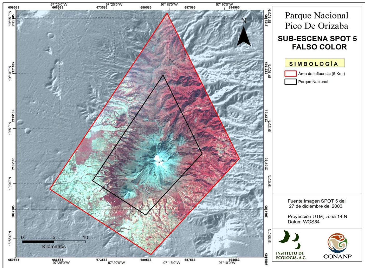
Figura 1. Sub-escena SPOT 5 del año 2003 en falso color (3, 2, 1).
