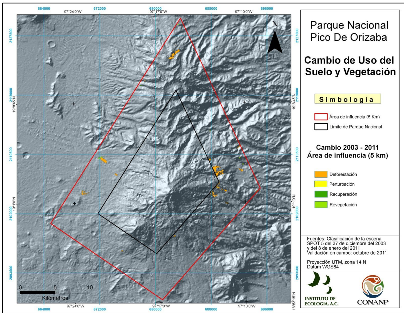
Figura 11. Cambios en el periodo 2003–2011 en el área de influencia (5 km al exterior del límite del PNPO).
