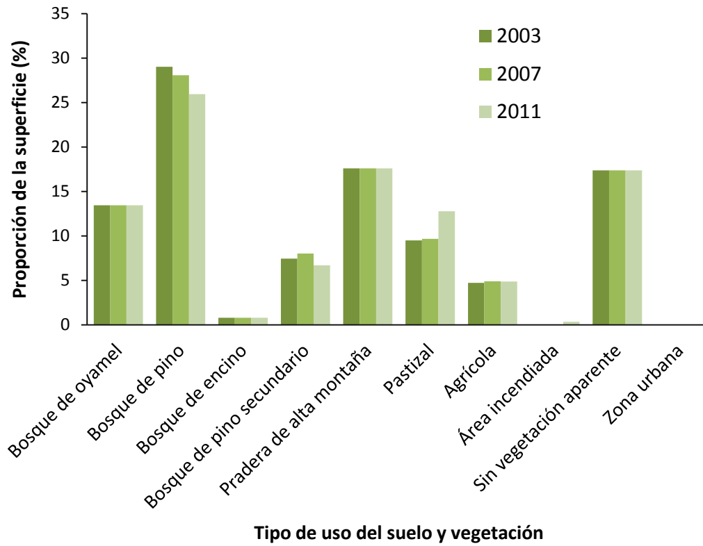
Figura 7. Proporción de la superficie (%) ocupada por tipo de uso del suelo y vegetación dentro del PNPO en cada fecha analizada.
