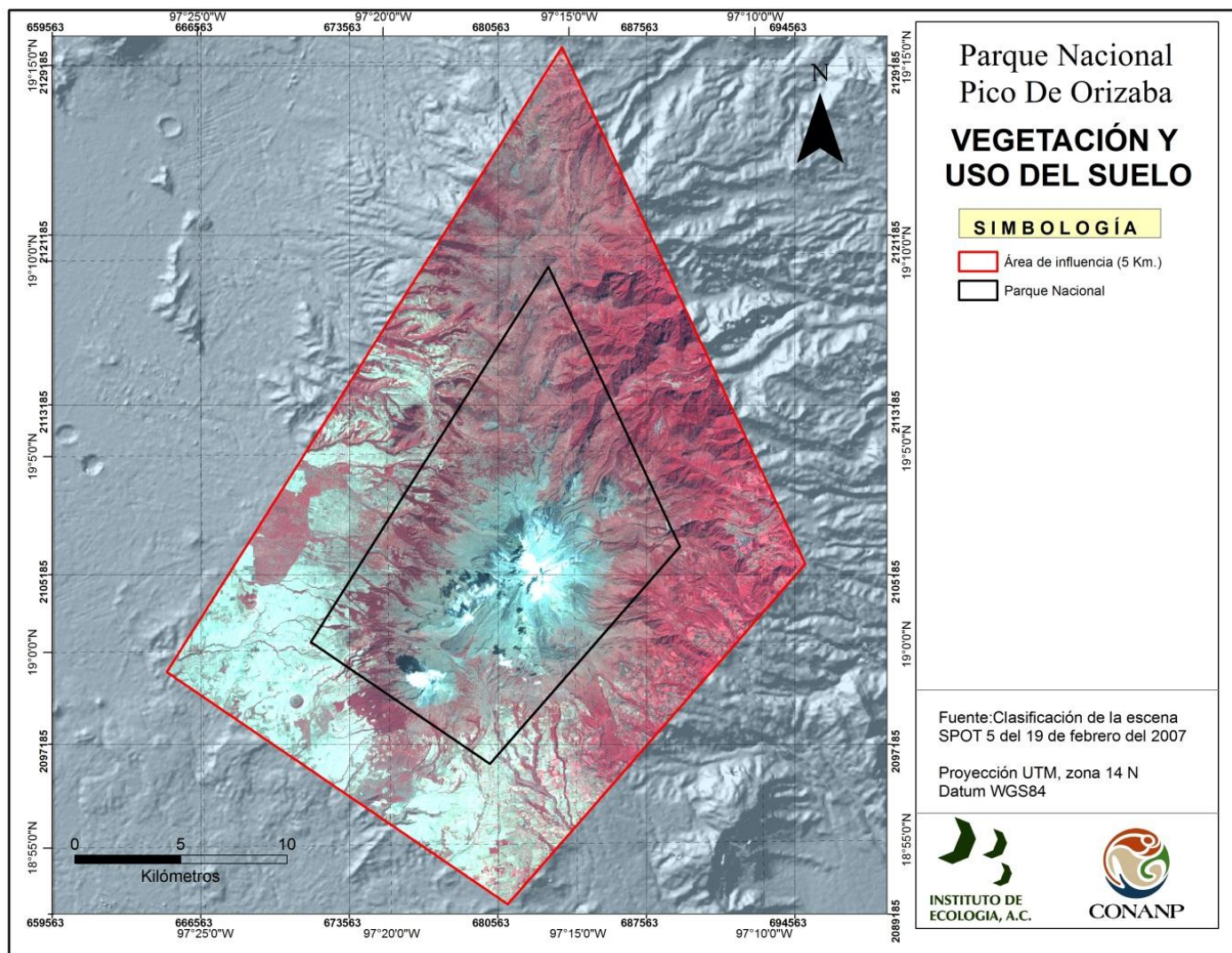
Figura 2. Sub-escena SPOT 5 del año 2007 en falso color (3, 2, 1).
